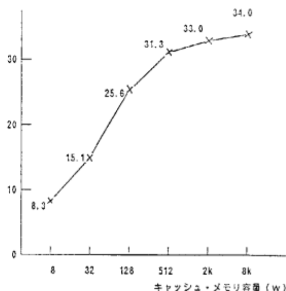
図 1 キャッシュメモリ容量と性能
