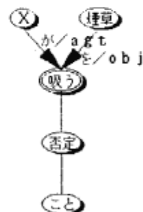
図4.13 「煙草を吸わないこと」の意味表現
