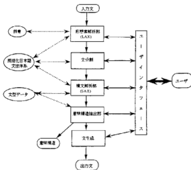
図2-1 ICOTEXTの処理概要
