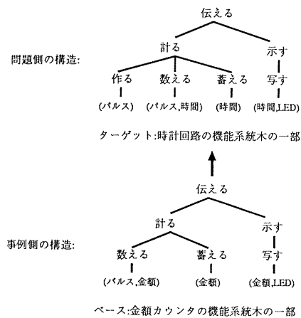
図2 SMEによる類似検索例
