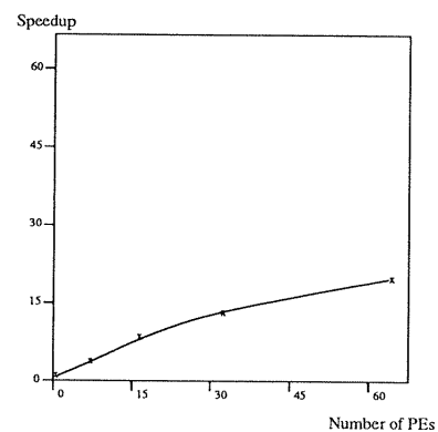
図3 並列検索による台数効果
